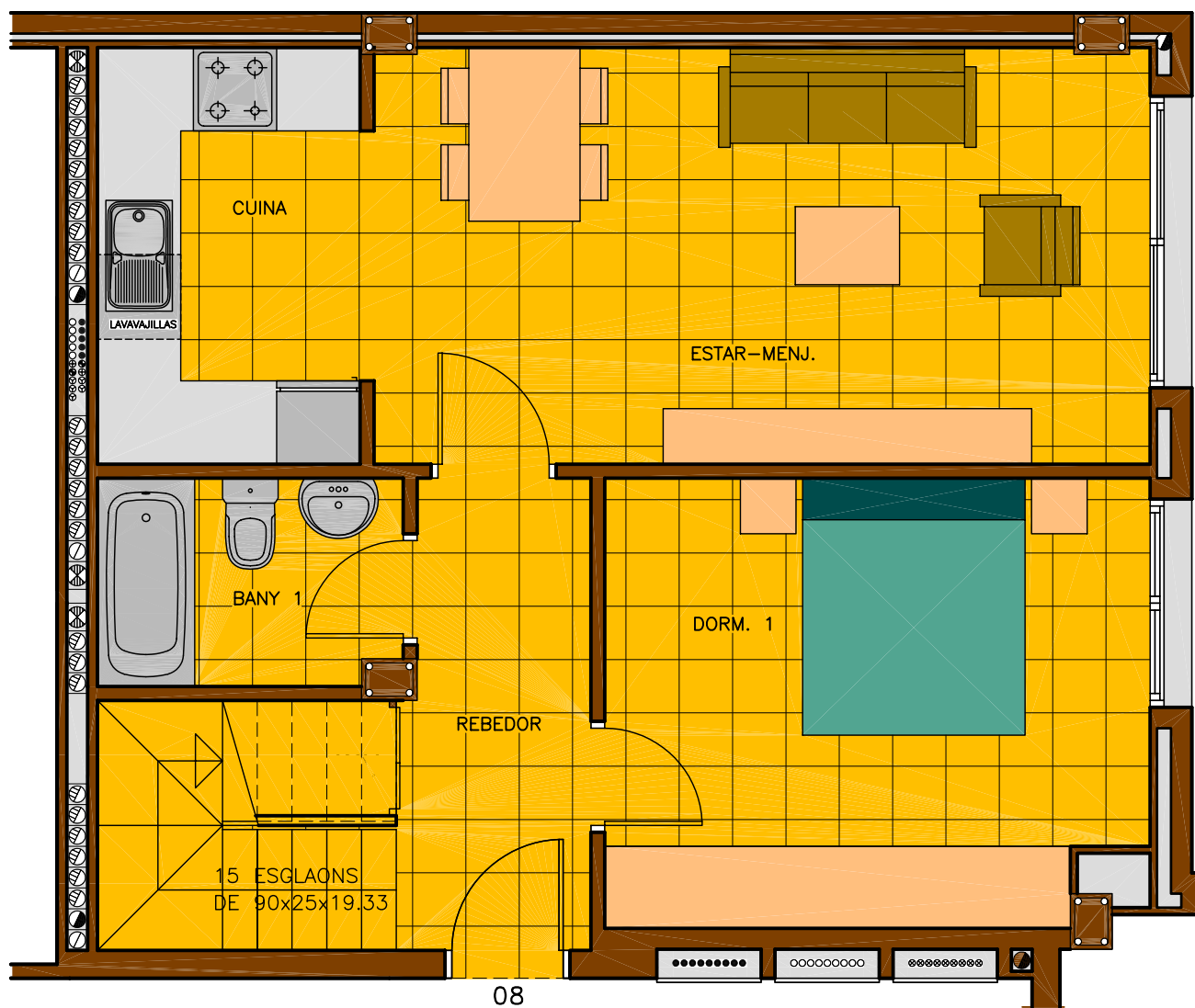
PLANTA 1º
